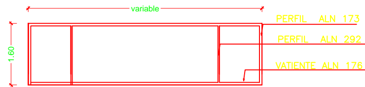
VENTANAS ALUMINIO SISTEMA PROYECTANTE 3831
