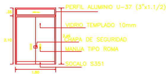
PUERTA ACCESO URGENCIAS
