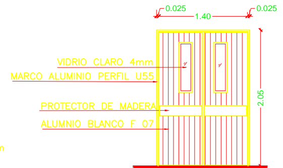
DETALLE PUERTAS TIPO VAIVEN ESC:1:20
