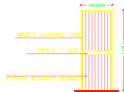
DETALLE PUERTAS TIPO ESC:1:20
