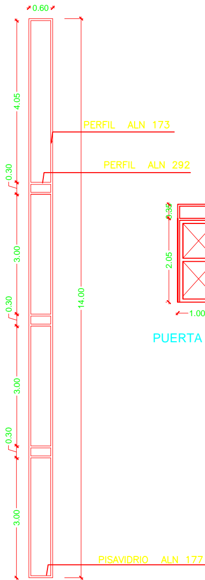
FACHADA FLOTANTE SISTEMA PROYECTANTE 3831
