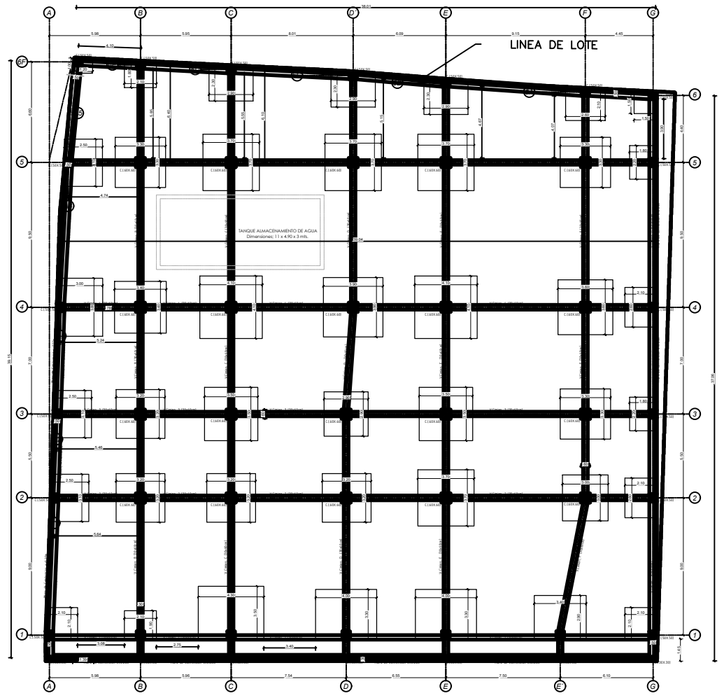
PLANTA DE CIMENTACION ESCALA: 1 : 75
