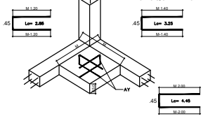
ZAPATAS ESQUINERAS
