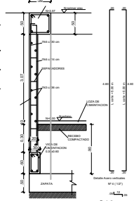
Detalle Muro en Ccto. Parquedero
