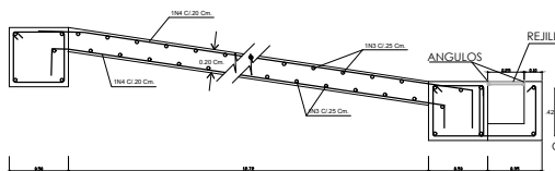
DET. RAMPA ACCESO SOTANO
